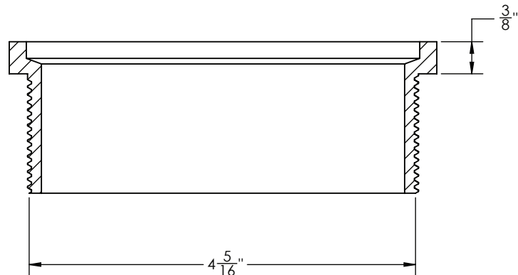
SECTION 1-1 SCALE 1 : 1
