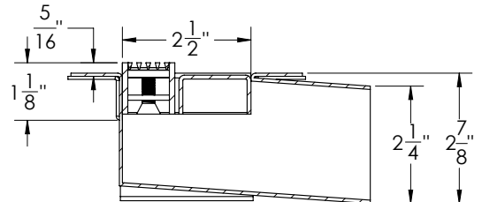
SECTION A-A SCALE 1 : 2
